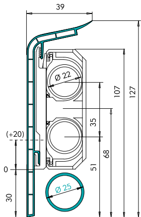
Maße des SLL Profils, hier mit Schelle Art.-Nr. 2250 und in Verbindung mit einem dritten Rohr
