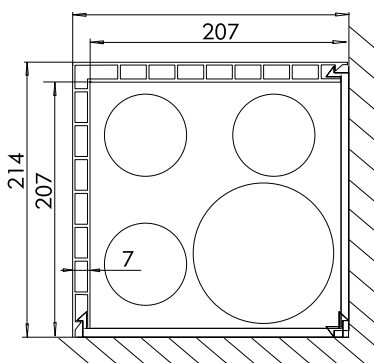
Maße des STP L 200 x 200 mm Art.-Nr. 6480
