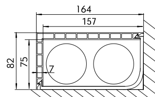
Maße des STP L 75 x 150 mm Art.-Nr. 6280
