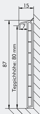
Maße der BLT
