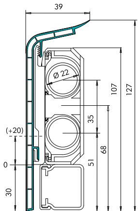
Maße des SLL Profils, hier mit Schelle Art.-Nr. 2250 und handelsüblichem Kabelkanal maximal 30 x 30 mm
