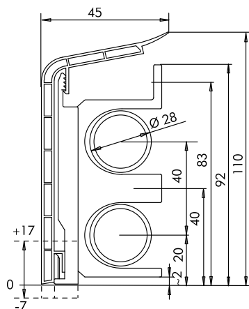
Maße des SLF 28 Profils und der Schelle Art.-Nr. 2450
