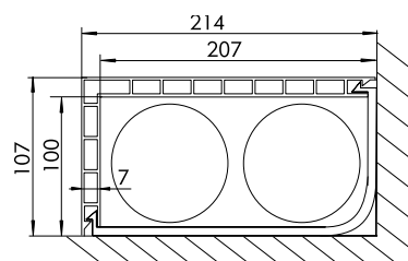
Maße des STP L 100 x 200 mm Art.-Nr. 6380
